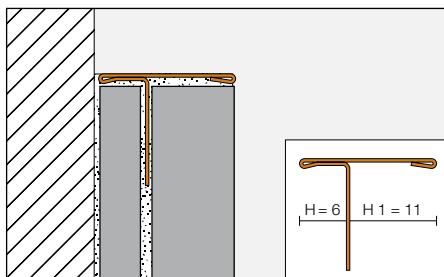
Příklad: Obklad na stávajícím obkladu se Schlüter®-SCHIENE-STEP-EB
